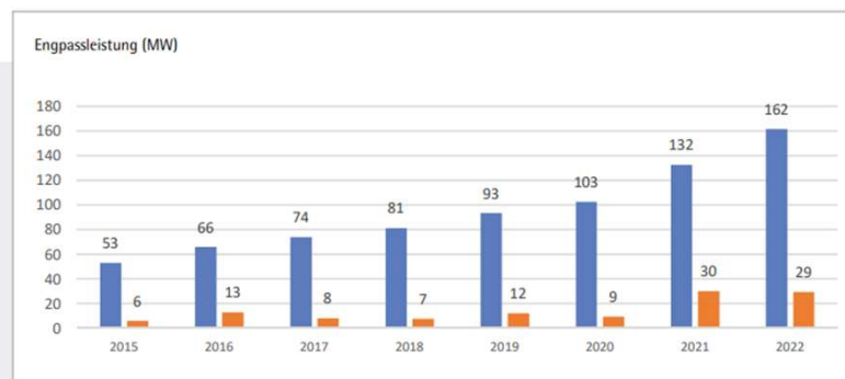
Engpassleistung Photovoltaikanlagen 2015–2022
