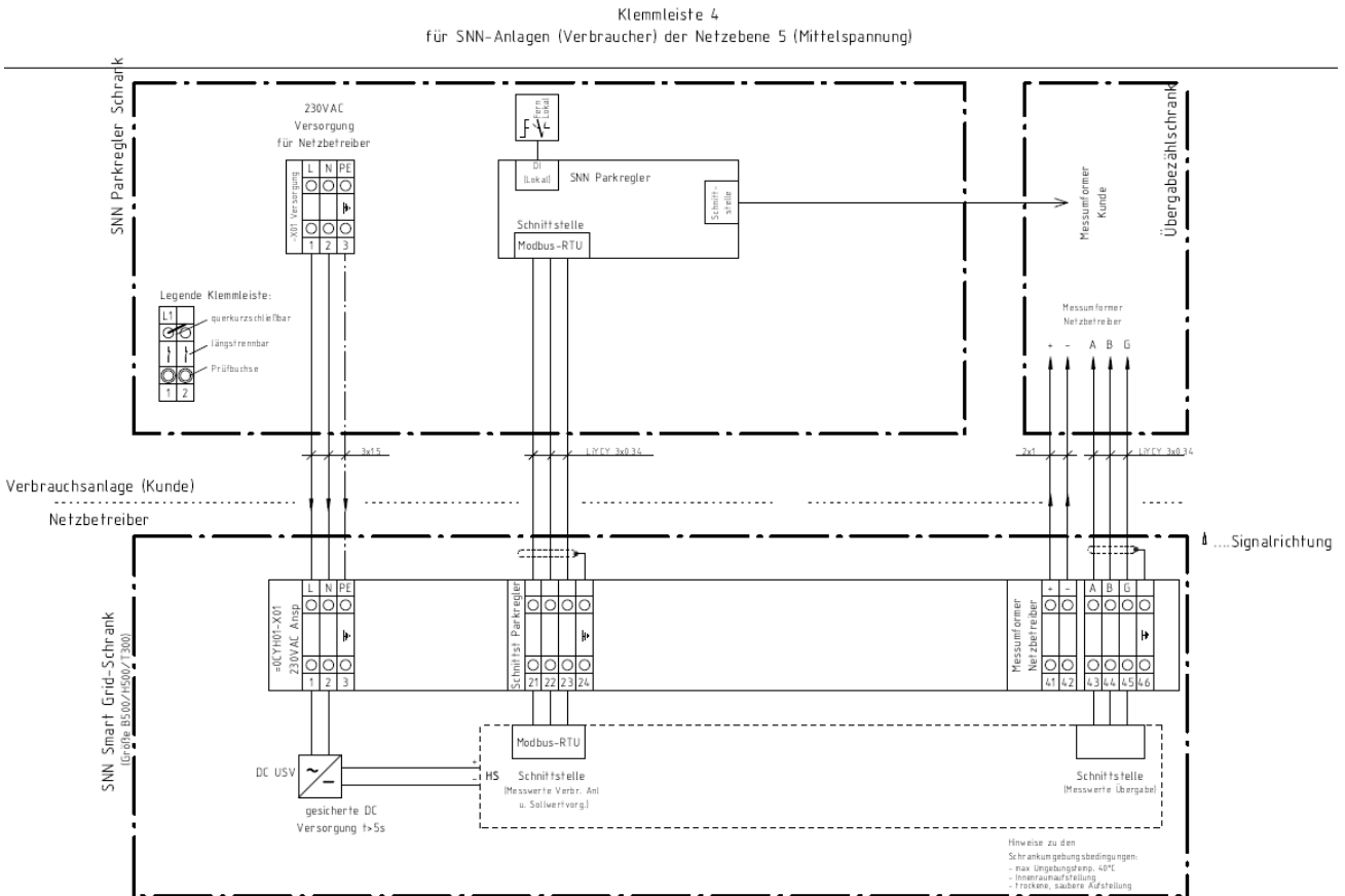
Abbildung 4: Klemmleiste 4 Modbus RTU Variante (P & Q) (Stand: Dezember 2023)
