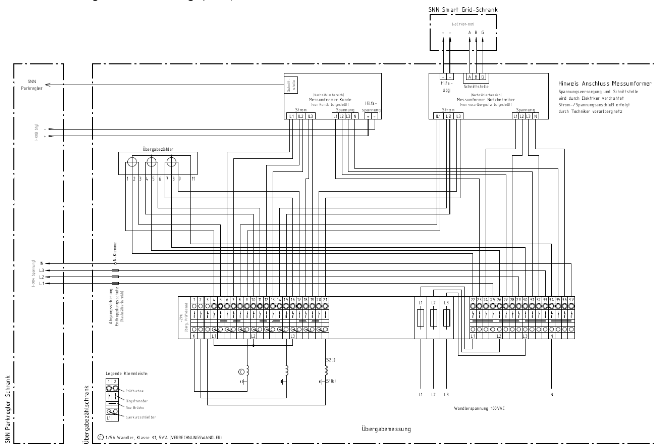
Abbildung 3: Klemmleiste Übergabemessung (MS) Stand: Dezember 2023
