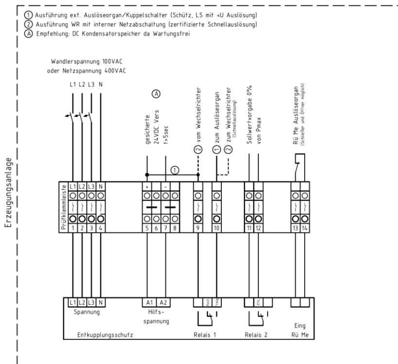
Abbildung 6: Klemmleiste 1 < 250 \text{ kW} (Stand: Jänner 2021)
