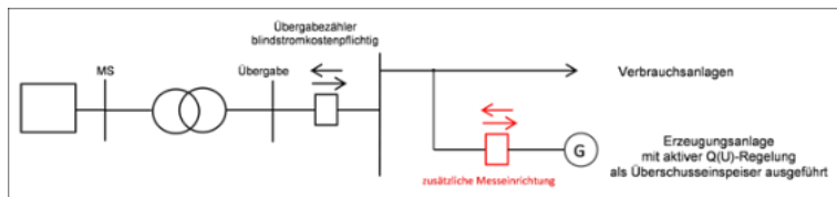
Abbildung 2: DEA-Messkonzept / Zähleranordnung
